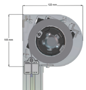
KASTENGRÖSSE 125
