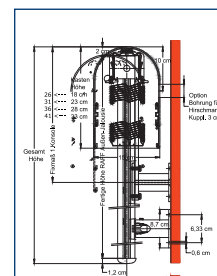
Voratzschacht rund
