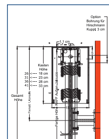
Voratzschacht eckig
